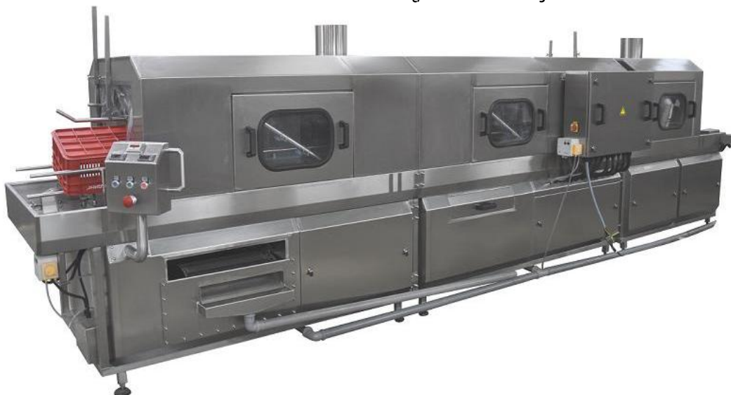
20.1316.32 – iki 600 dėžių, su būgniniu filtru, skaitliukas išplautoms dėžėms, flanšas
